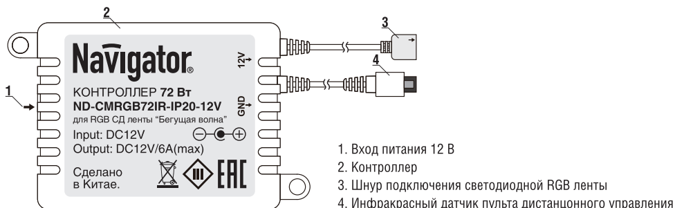
Рис. 1. Схема контроллера.
