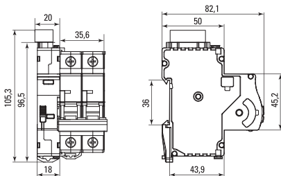
Рис. 3 Габаритные размеры моторного привода
