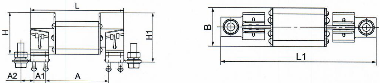
Рис. 1. Общий вид
