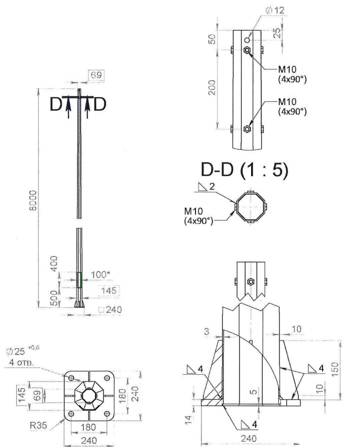
Рис.1 - Габаритные и присоединительные размеры
