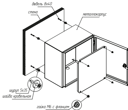
Рис. 1.1 - Схема настенного монтажа
