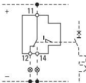
Рис. 1 Схема подключения
