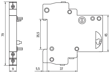
Рис. 2 Габаритный и установочный размеры БК
