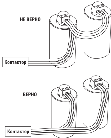
Рис. 3 – Параллельное подключение конденсаторов
