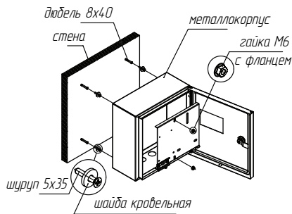
Рис. 1.1 - Схема настенного монтажа
