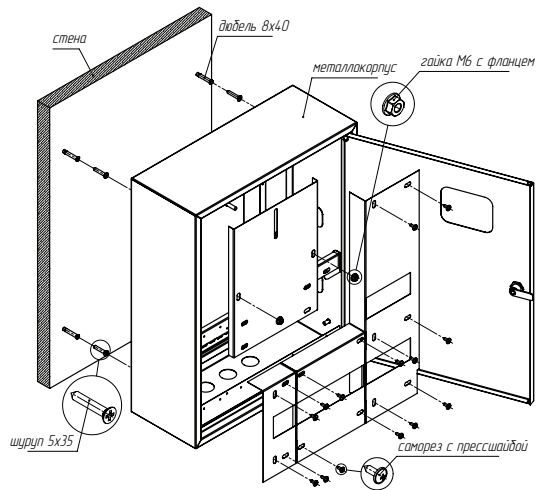
Рис. 1 - Схема монтажа
