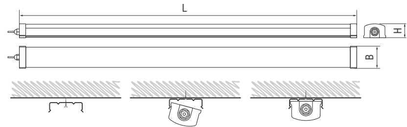
Рис.1 Схема монтажа светильника PWP-C3
