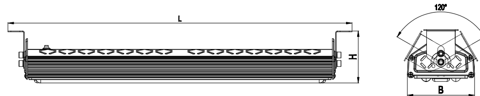
Рис. 1 Светильник PPI-04
