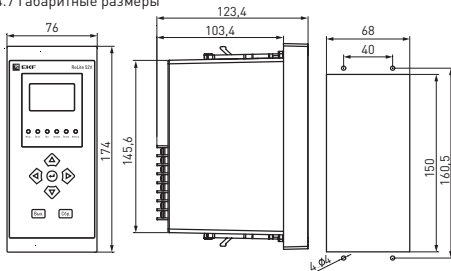
Рис. 3 – Габаритные размеры устройства ReLite 52 в вертикальном исполнении
