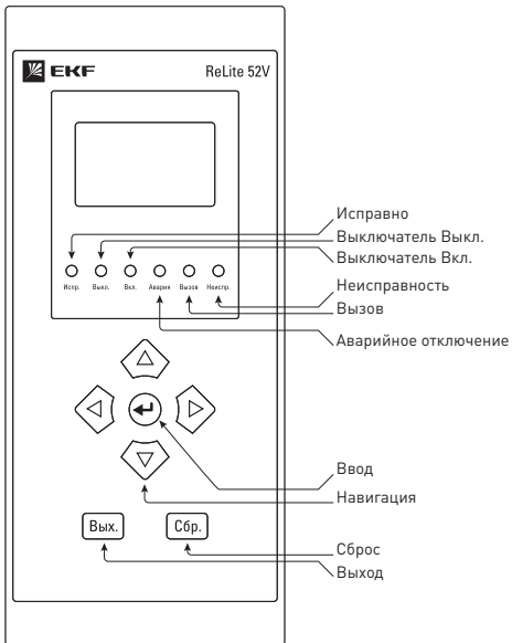
Рис. 1 – Лицевая панель ReLite 52
