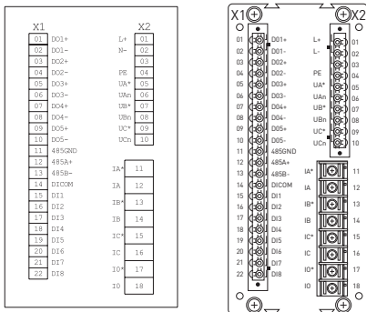
Рис. 2 – Расположение клемм
