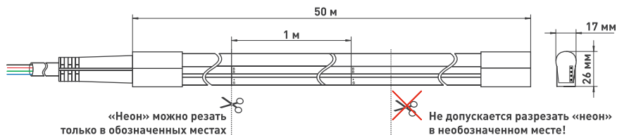
Рисунок 1. Габариты ленты «гибкий неон».
