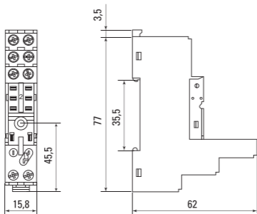
Рис. 6 - Габаритные размеры PM5 22/2 EKF AVERES
