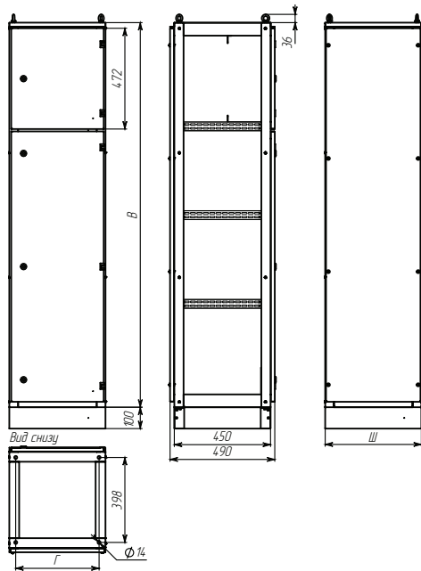
Рис.1 - Общий вид шкафов ВРУ-2 Unit S
