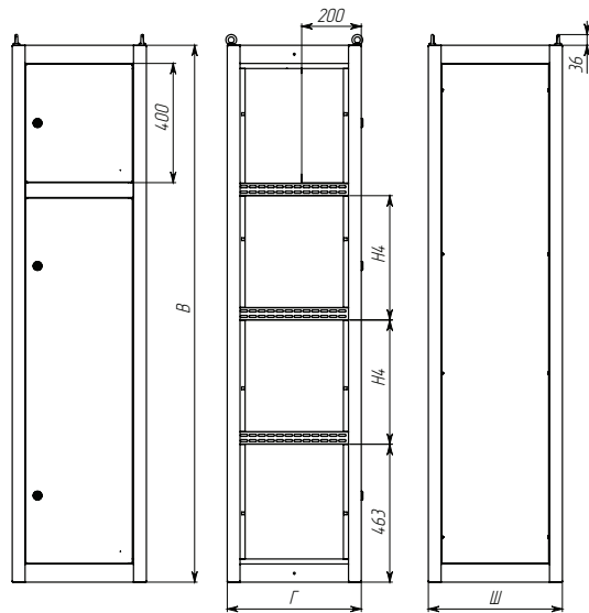
Рис.1 - Общий вид шкафов ВРУ-2 Unit S
