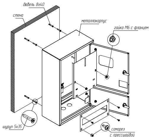
Рис. 1 - Схема монтажа
