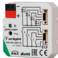
025679 KNX-309-4DRY-IN
