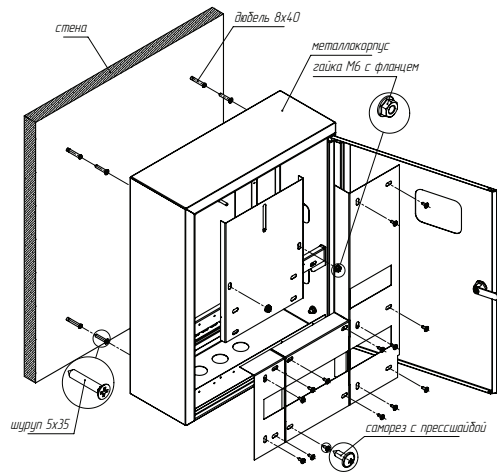
Рис. 1 - Схема монтажа
