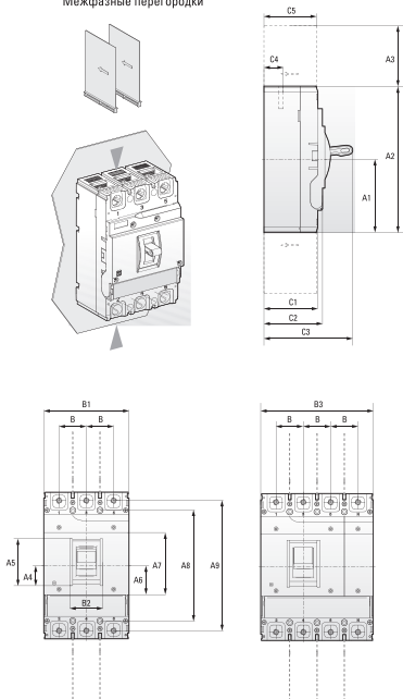
Рис. 3 Габаритные размеры AV POWER-1 (2) (3) (4)
