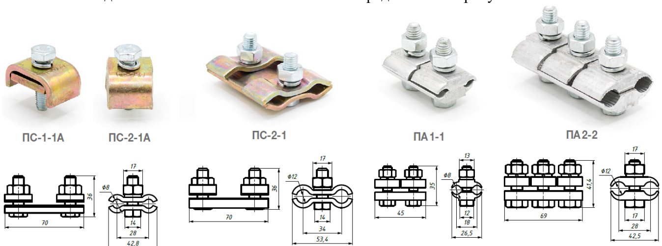
Рис. 1. Внешний вид плашечных зажимов типа ПС и ПА.
