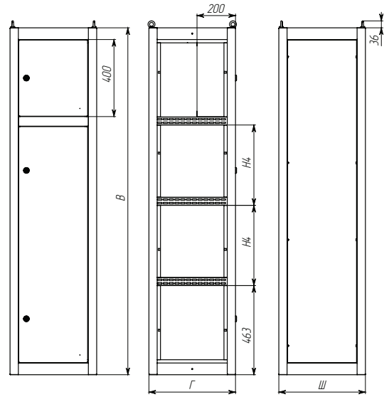
Рис.1 - Общий вид шкафов ВРУ-2 Unit S
